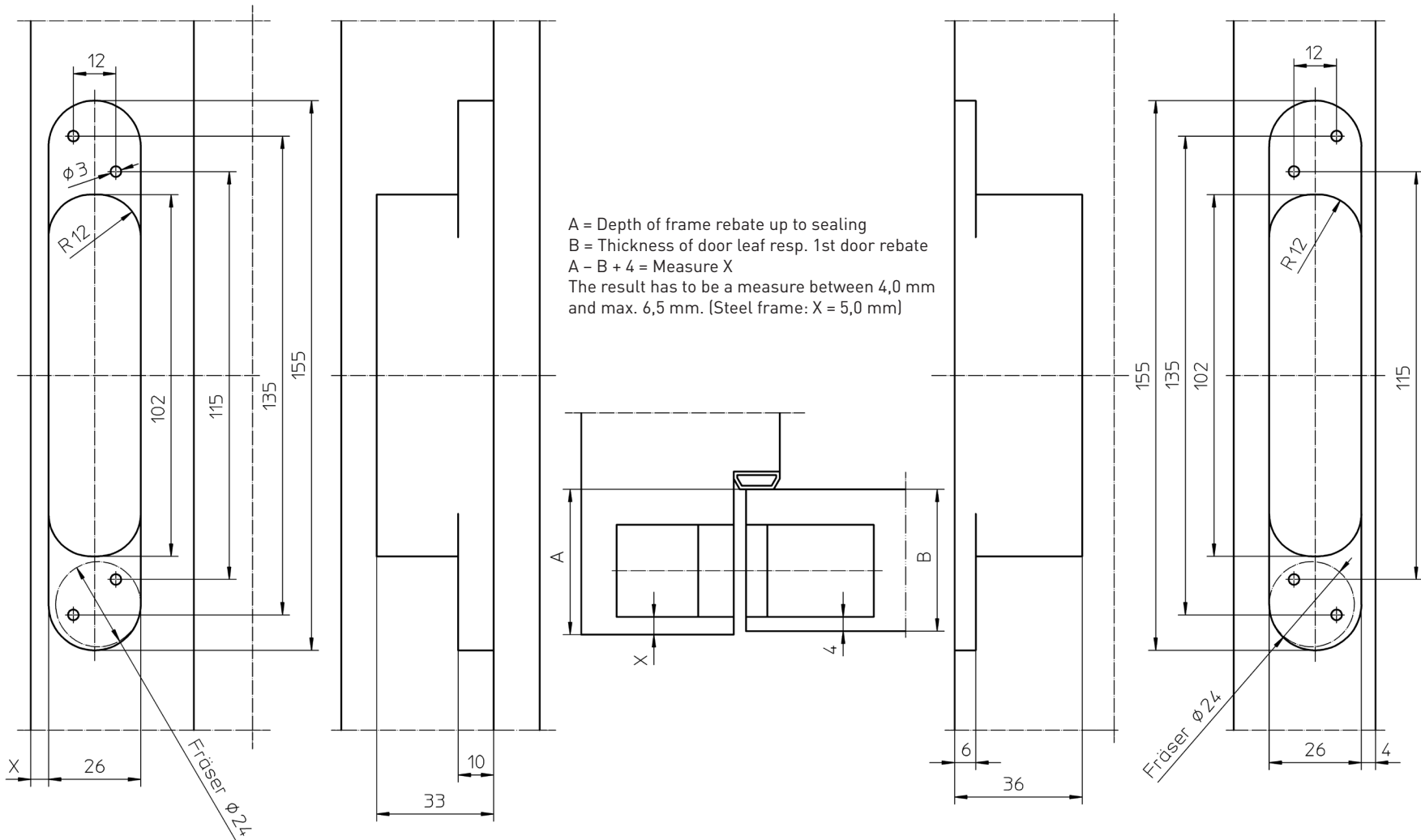
MILLING : DOOR LEAF
